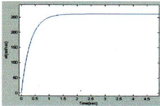
Gambar 16. Hasil Simulasi kendali motor dc dengan I_f berubah dan asumsi I_a konstan ( \omega \propto V_s t )
